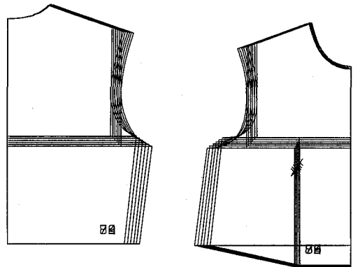
図4 Bust 寸法2 cm ピッチのグレーディング (B=74 cm から84 cm の6 サイズ)
